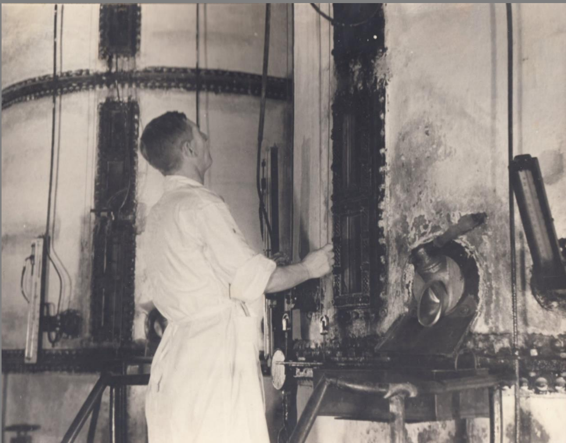
Vakumaparāti, kur iegūst 1., 2., 3. šķiras cukuru
